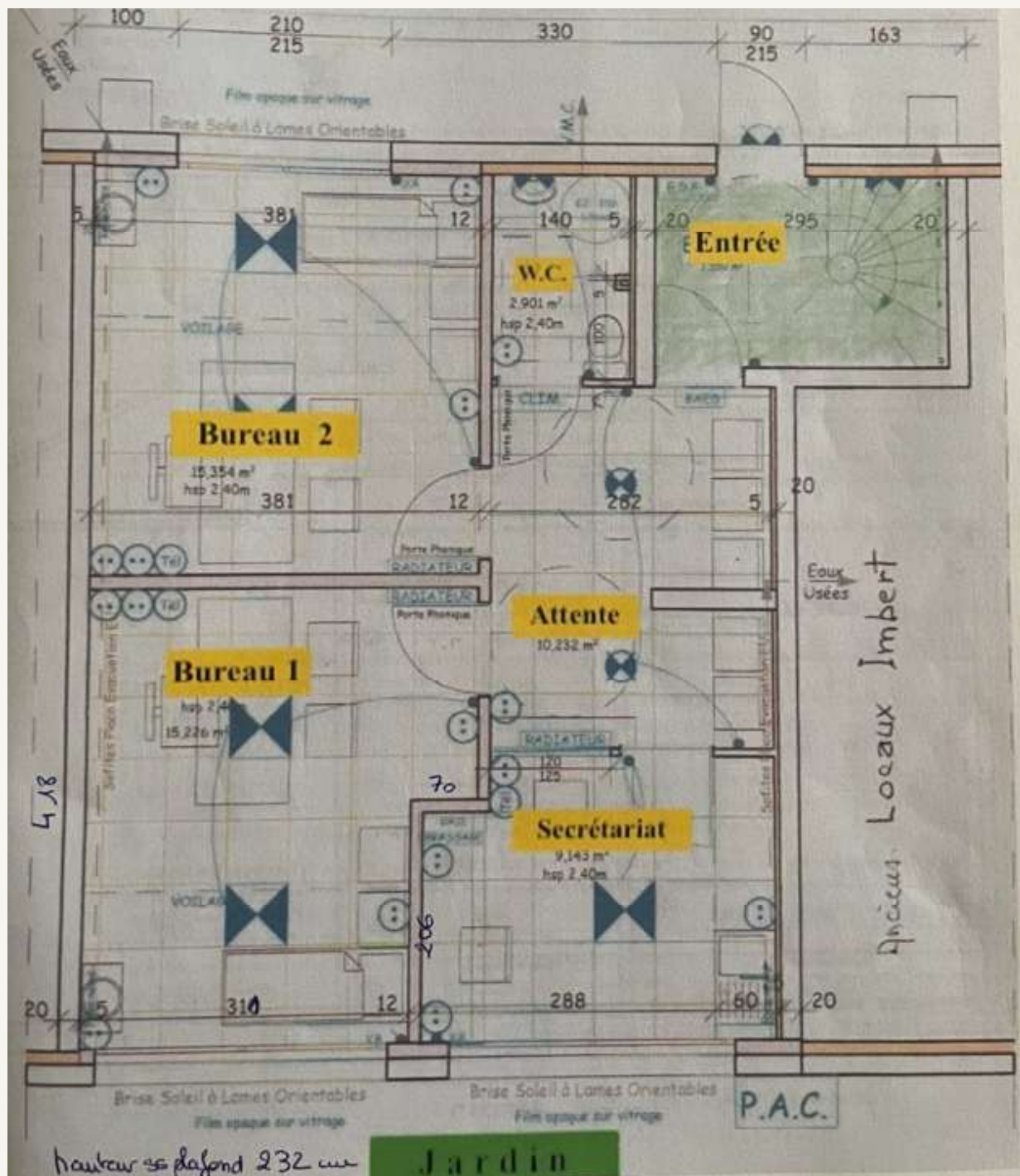
Plan du rez-de-chaussée
